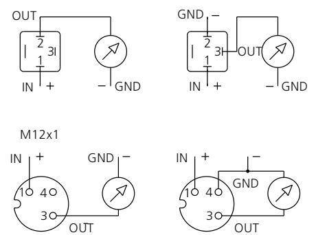
Fig. 2 Connector DIN 175301-803-C (mini DIN)
