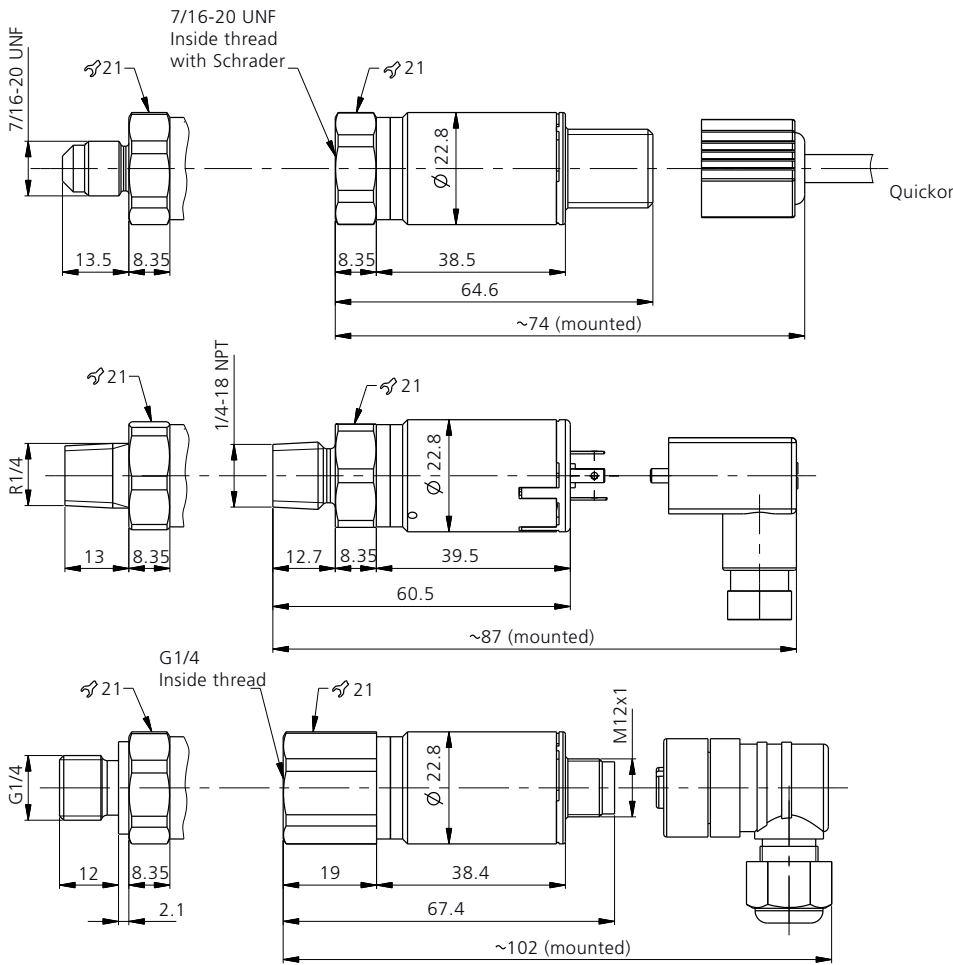
Fig. 1 Connector DIN 175301-803-C (mini DIN)
