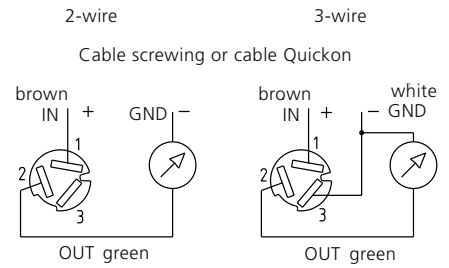
Fig. 1 Connector DIN 175301-803-C (mini DIN)
